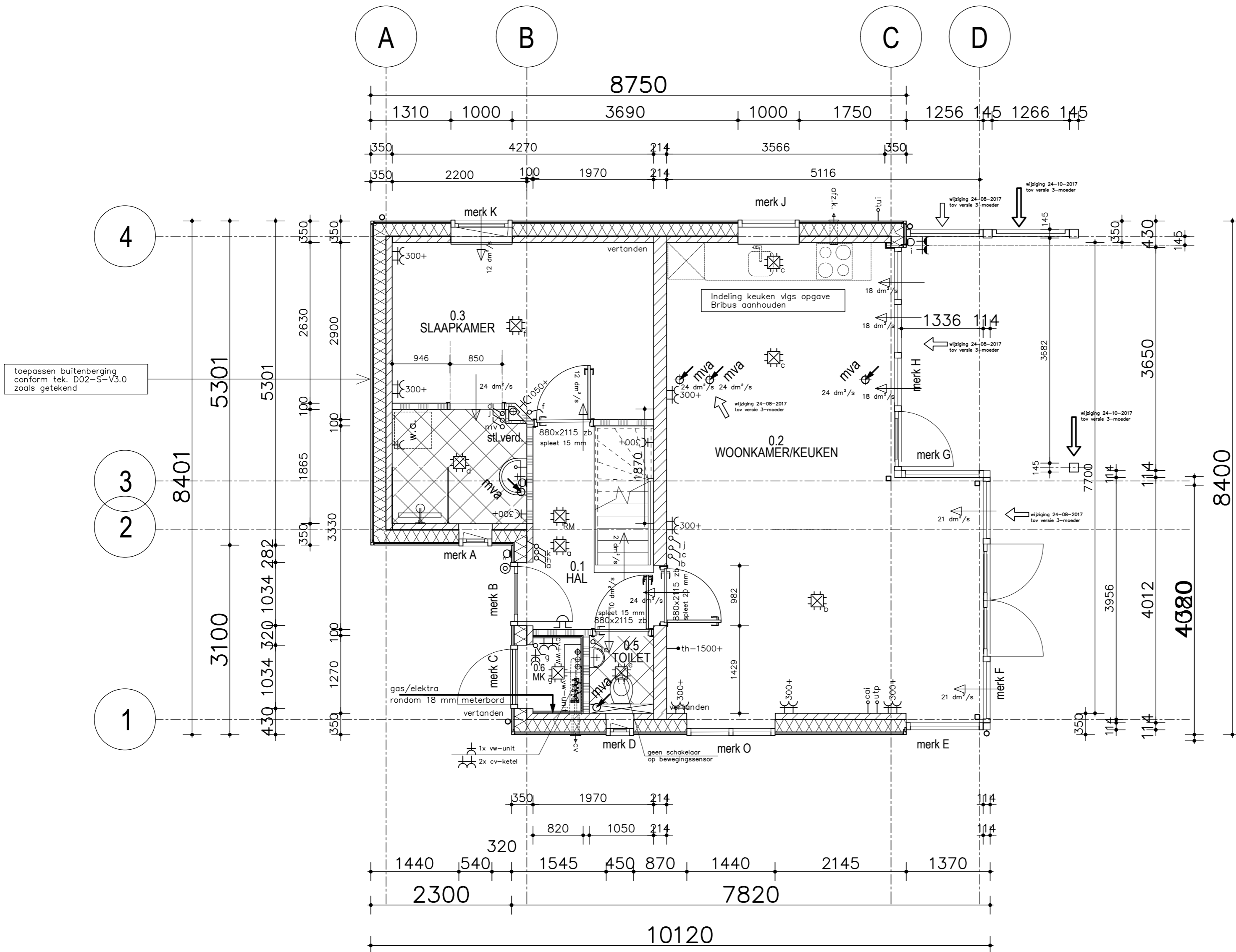
plattegrond begane grond
